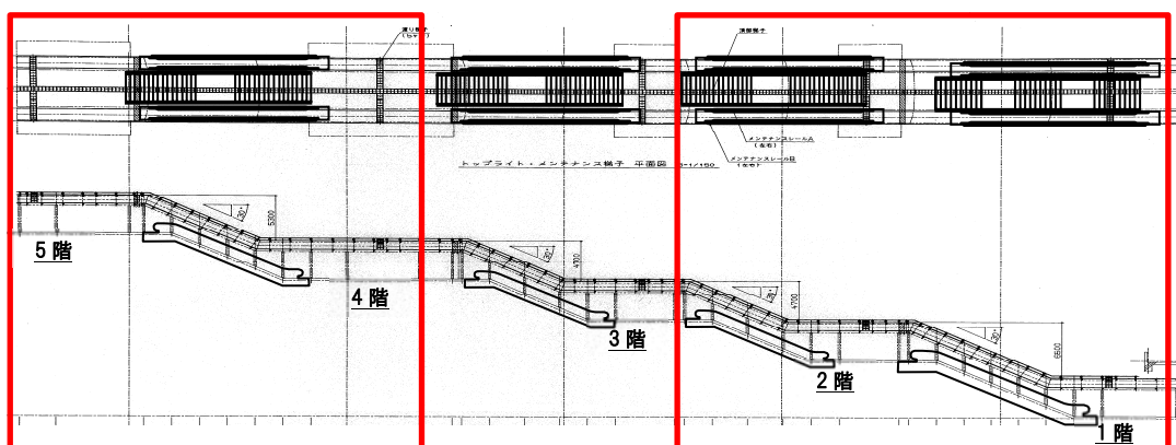
エスカレーター (4階～5階 平日夜間22:00～翌7:00閉鎖)
