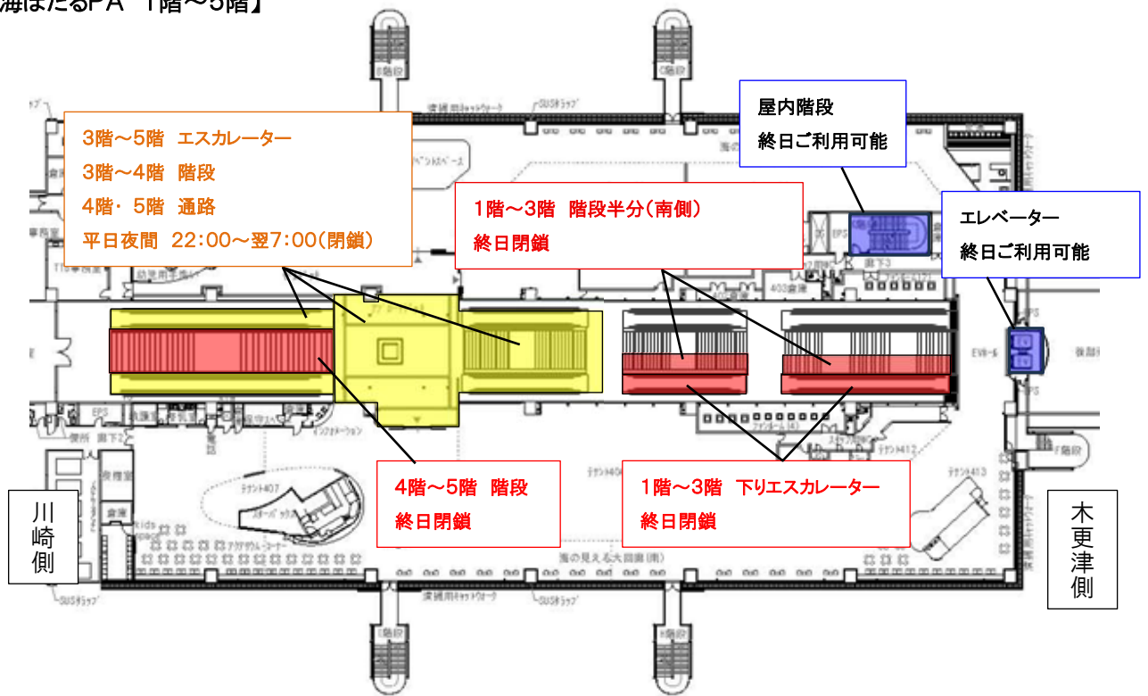
下りエスカレーター(1階～3階終日閉鎖)
